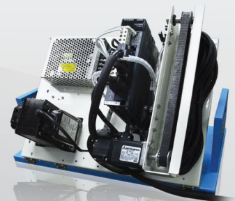
TW-NC1 370x430x310mm
